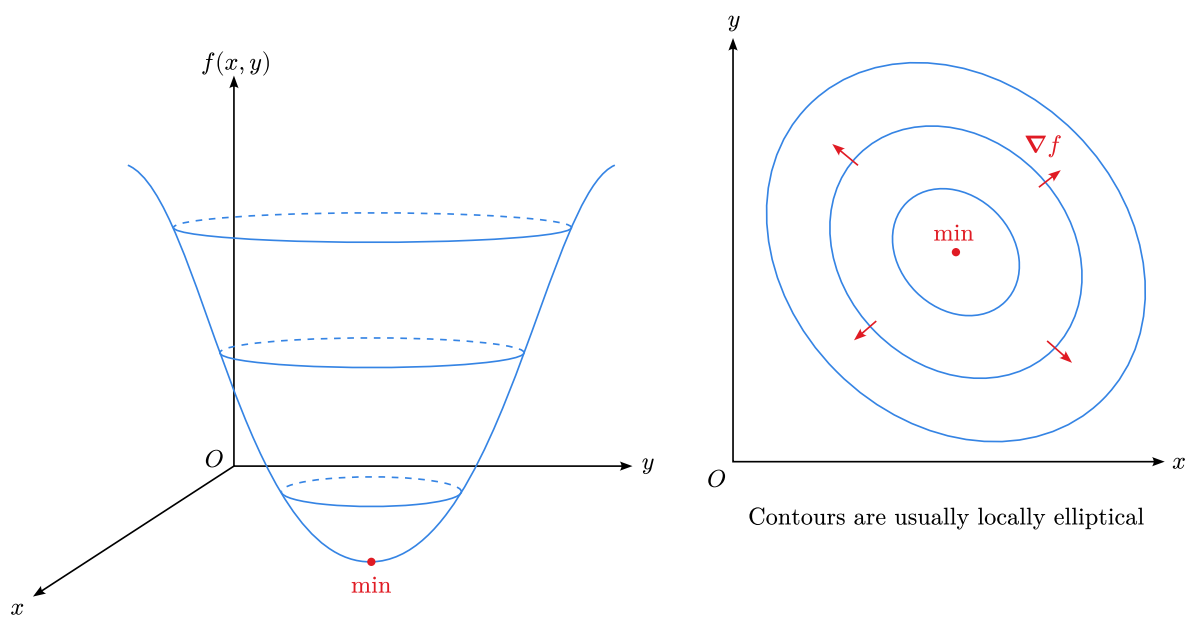
Local Minima
